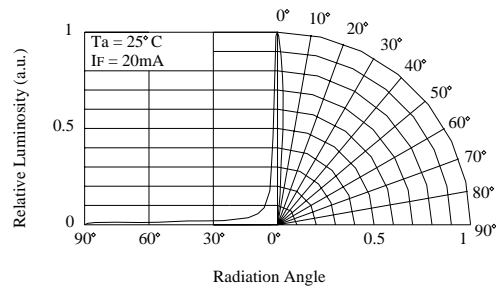
Directivity (Angle : 8°)
