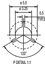
P DETAIL 1:1
