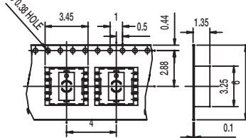
P DETAIL 1:1
